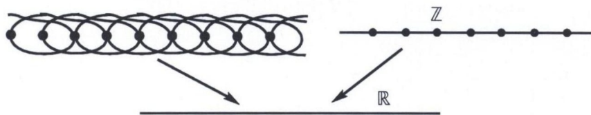
Figura 1: El grafo de la derecha corresponde a \{1\} , el de la izquierda a \{2, 3\} . Ambos grafos, vistos desde el infinito, se convierten en una línea.
