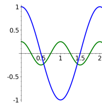
Gráficas de coseno
