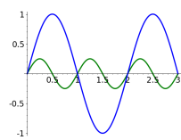
Gráficas de seno
