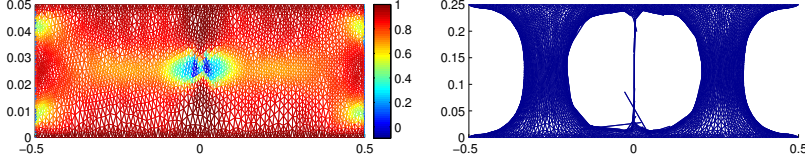
FIG. 6.3. A thinner bar: (-0.5, 0.5) \times (0, 0.05) , \lambda = 5 .
