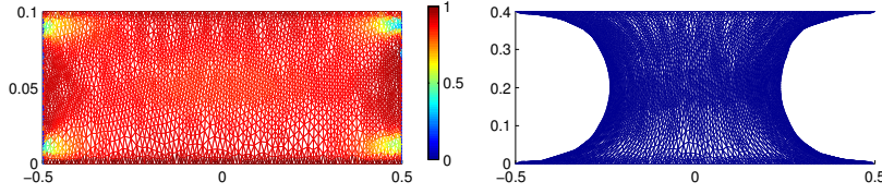
FIG. 6.1. A bar: (-0.5, 0.5) \times (0, 0.1) , \lambda = 4 .
