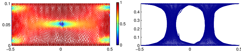
FIG. 6.2. A bar: (-0.5, 0.5) \times (0, 0.1) , \lambda = 5 .
